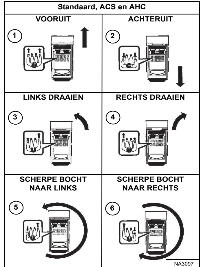
Functies van de stuurhendel (rijden en sturen) [Figuur 60]
